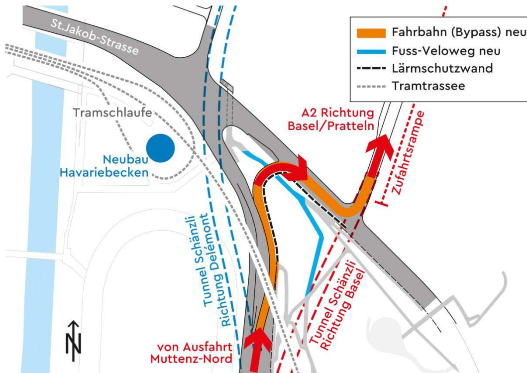
Grafik Nr. 1: Provisorische Verkehrsführung Bypass (13.10.2017 - Feb. 2021) (Quelle: www.epschaenzli.ch/verkehrsuehrung/umleitung )
